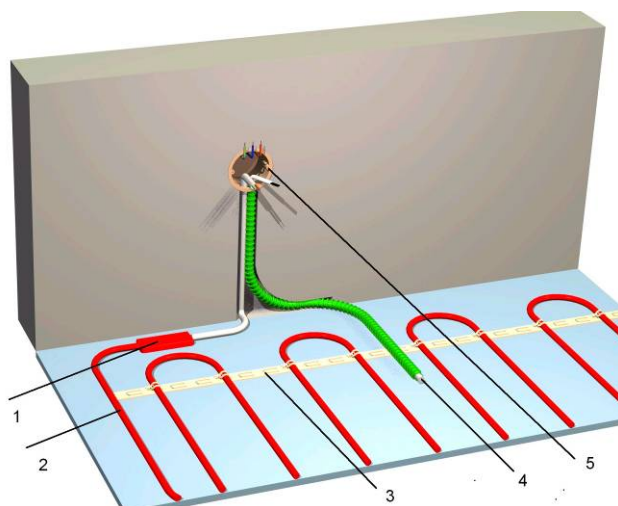
Рис. 3. Монтаж датчика температуры в системе “Теплый пол”.
