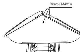
Рис. 12 – Установка козырька
