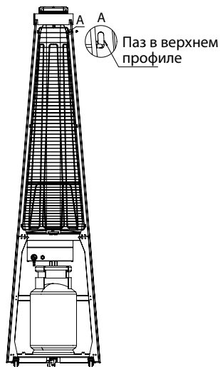
Рис. 10 – Установка фиксаторов решетки
