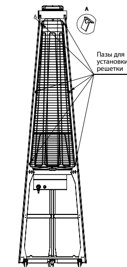
Рис. 9 – Установка решетки
